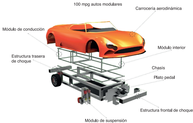
Figura 2. Diseño modular Wikispeed.
