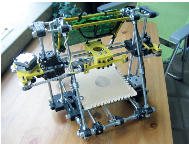
Figura 1. Rep Rap v.3 (Huxley), Licencia GPL 2.0. Mayo 2007.
